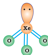
(e) Pyramidal
