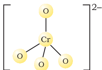
Chromate ion
